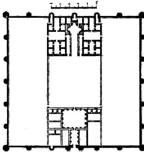
(تخطيط ١٨) : قصر مشتى جنوب شرقى عمان (الأردن) من حوالى ١٢٧- ١٣٣هـ/٧٤٤-٧٥٠م . عن: فريد شافعى : العمارة العربية ، شكل ١٧٣ ص ٢٥٢ .)
